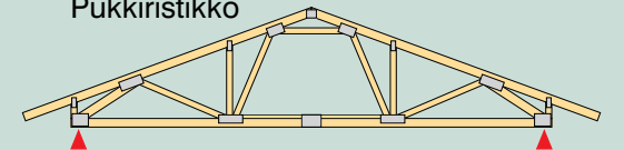
Käyttöullakkoristikko
